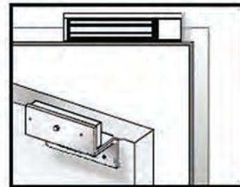
LZ-bracket for inswing door
