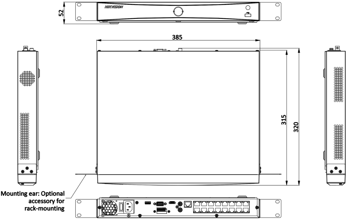
scale/1:1;Unit/mm
